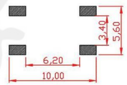
PCB. 焊接图
