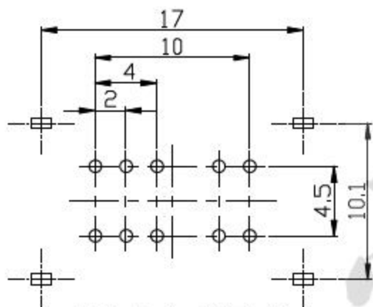
P.C.B LAYOUT
