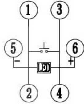
电原理图
