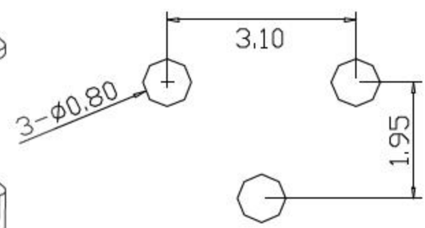
PCB. 焊接图
