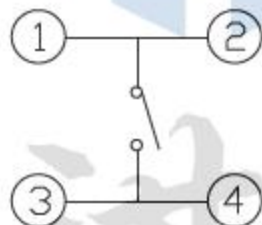
电路图
