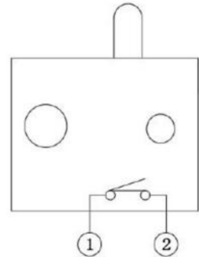
电路图：常开式(N.O) 1个电路1个接点 端子排列（自A方向看）
