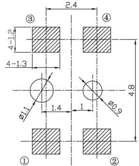
安装位置图
