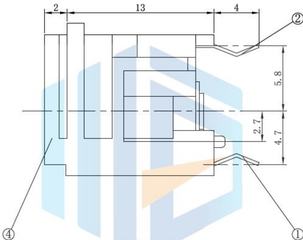
接点示意图
