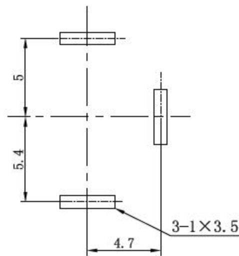
印制电路板开孔尺寸
